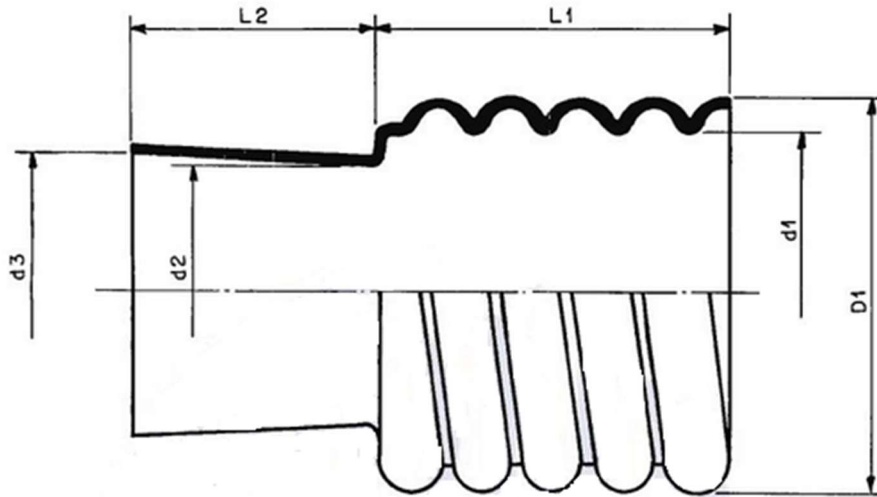
Figura 1 – Conexão II para união de dutos
